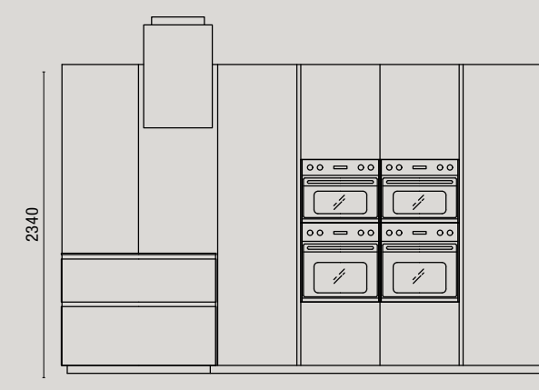
PROSPETTO C-C Front view C-C
