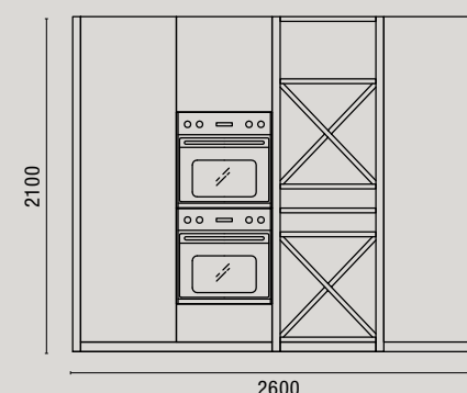
PROSPETTO E-E Front view E-E
