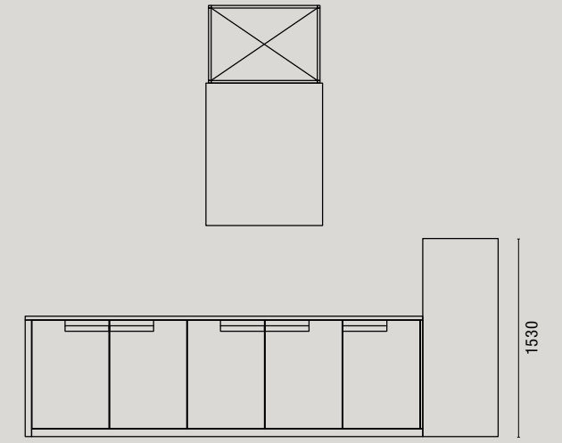
PROSPETTO B-B Front view B-B
