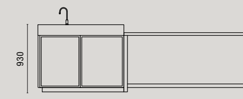
PROSPETTO B-B Front view B-B
