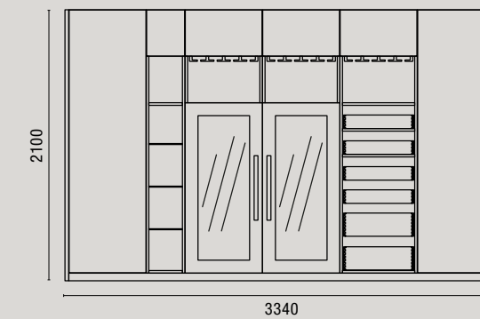
PROSPETTO F-F Front view F-F
