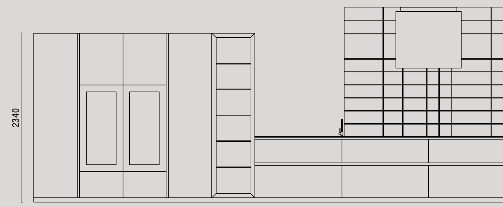
PROSPETTO A-A Front view A-A
